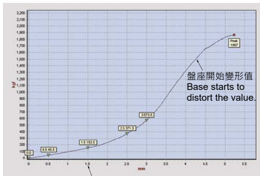
設定荷重 150 kgf 下壓值 1.5 mm，合金鋼 Ø40圓腳 座荷重測試曲線圖
