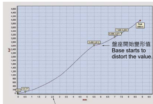
設定荷重 700 kgf 下壓值 2.5 mm，不鏽鋼304 Ø90 圓腳座荷重測試曲線圖
