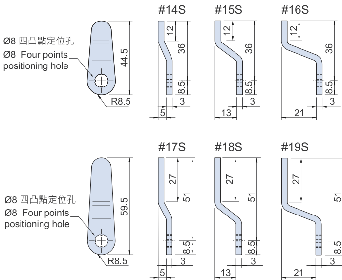
檔片型式 Pawl Type
