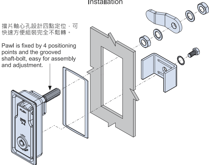
裝配示意圖 Installation
