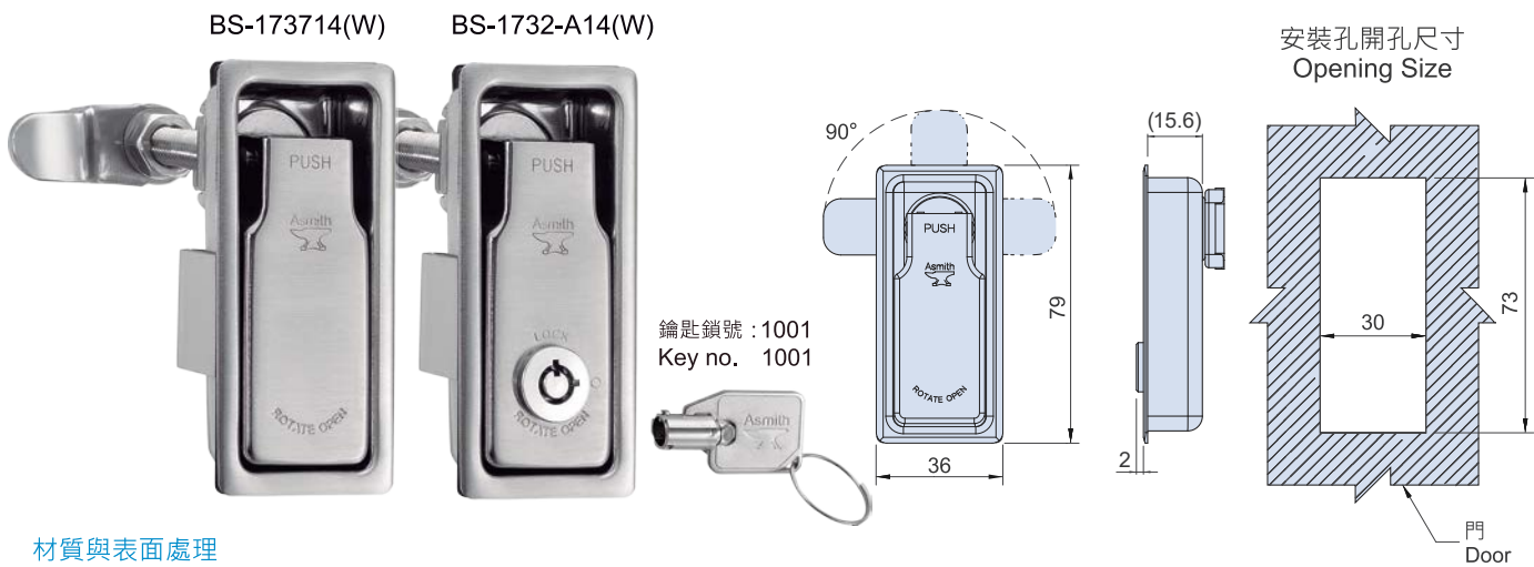
裝配示意圖 Installation
