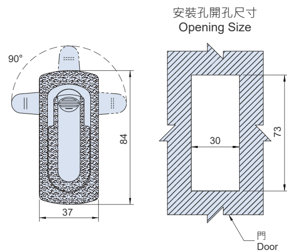
裝配示意圖 Installation
