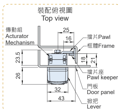
安裝示意圖 Installation
