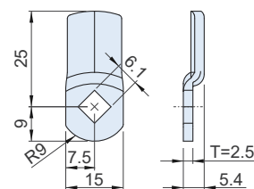
擋片 Pawl
