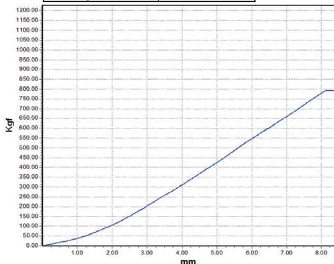
CS-5230 調整搭扣荷重測試曲線圖 The chart shows the Draw Latches (Adjustable Type) load capacity of CS-5230
