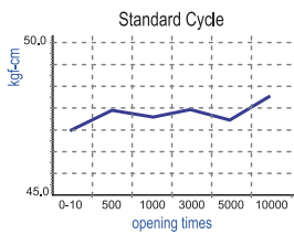
AZ-0620-47開合次數與扭力變化
