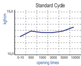
AZ-0621-12開合次數與扭力變化
