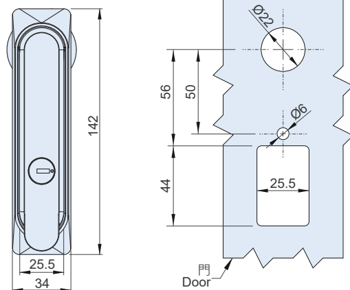
安裝孔開孔尺寸 Opening Size
