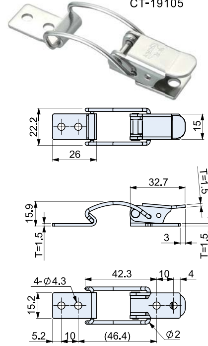
CS-19105 CT-19105
