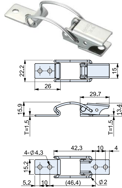
CS-19102 CT-19102
