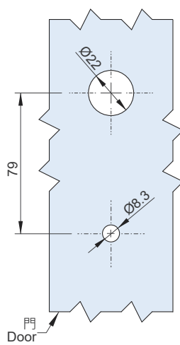
安裝孔開孔尺寸 Opening Size
